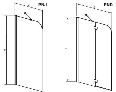
Lavostranné prevedenie vaňovej zásteny
